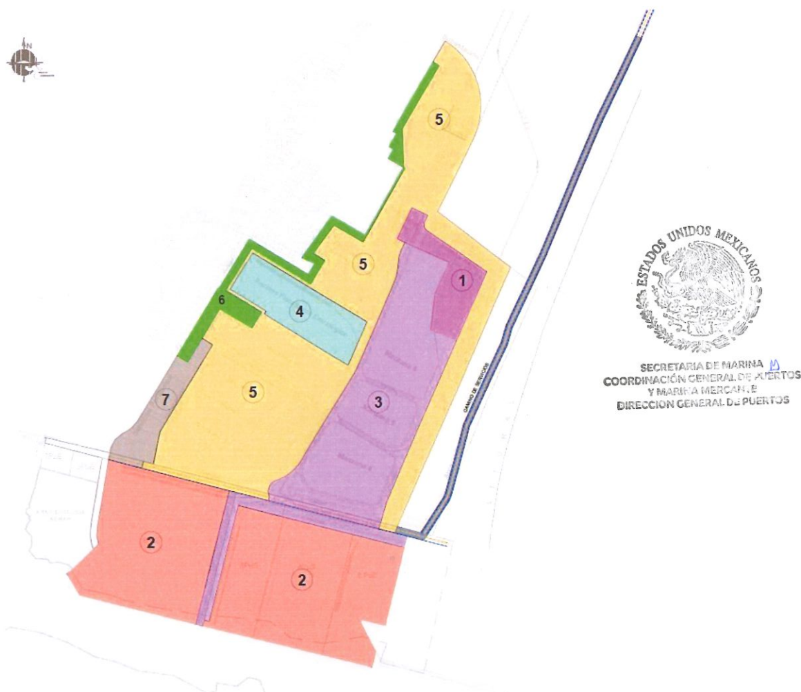
Plano de zonificación general del Puerto de Matamoros y sus ZDP Elaboración propia.
