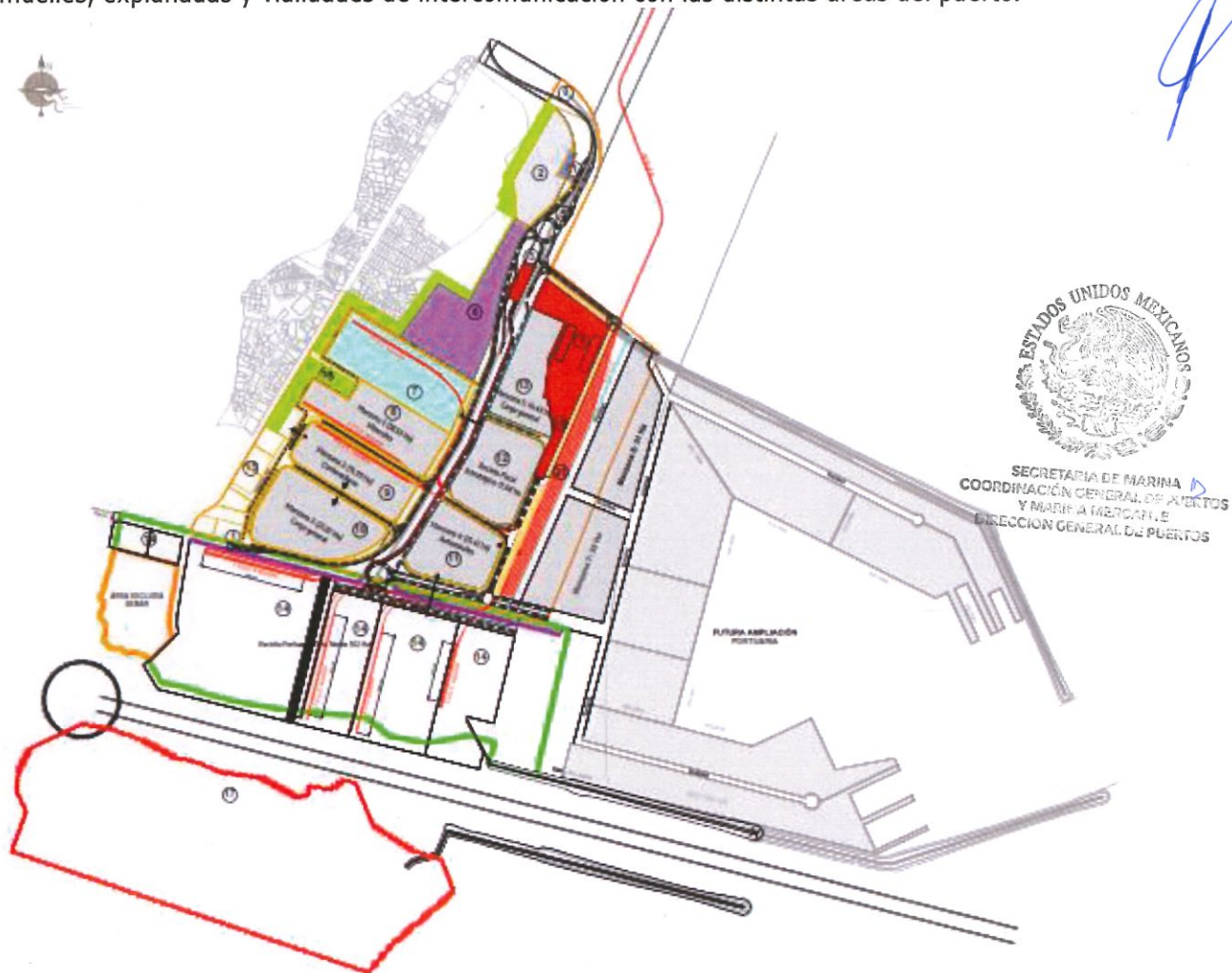
Imagen de la etapa 3 de largo plazo con el proyecto conceptual de construcción de nuevos rompeolas y muelles en la zona noreste del Puerto de Matamoros.
