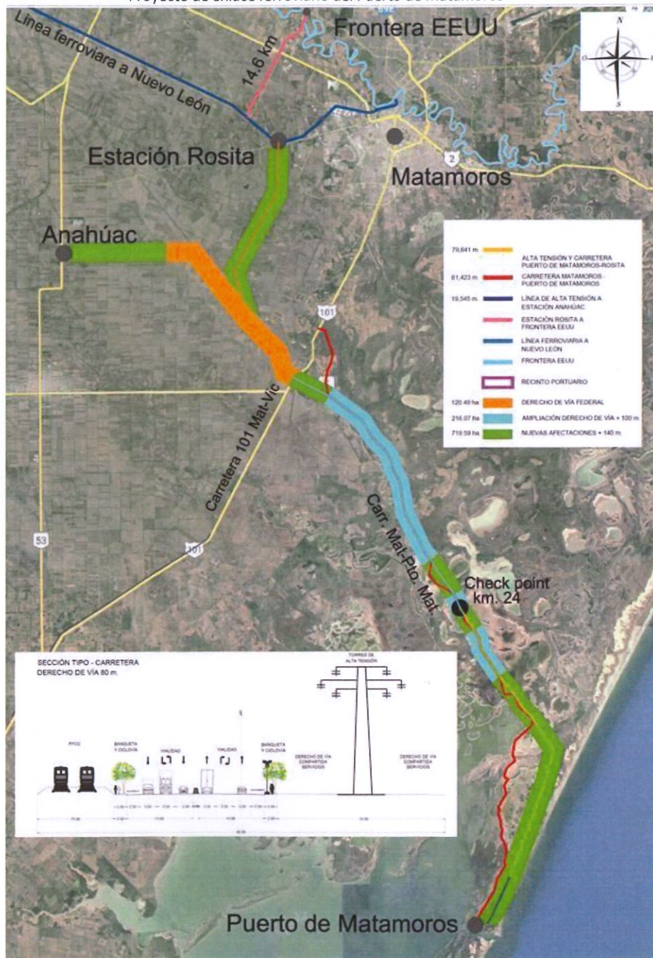
Proyecto de enlace ferroviario del Puerto de Matamoros
