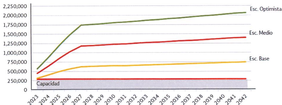
Comparativo de oferta y demanda de granel mineral en el Puerto de Matamoros, 2023-2042 (toneladas)
